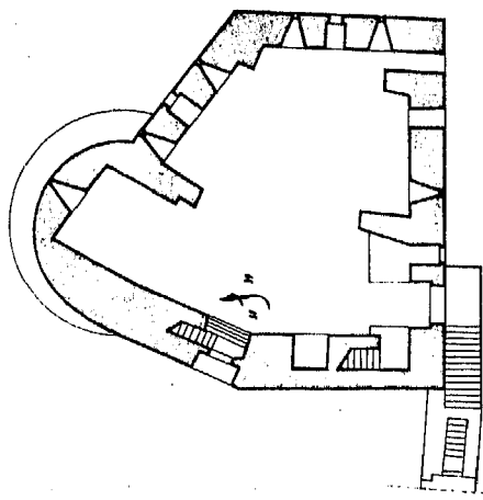
تخطيط للبيج الملوكي مقياس ١/٤٠٠
